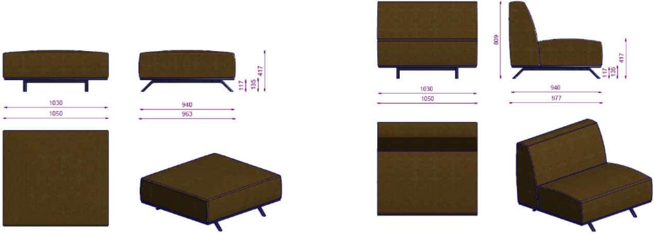
OSCAR S0 105 PUF w:1050 d:963 h:415 mm
