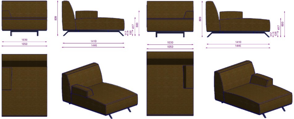
OSCAR S0 105 SOL UZAN KLTK w:1050 d:1446 h:807mm
